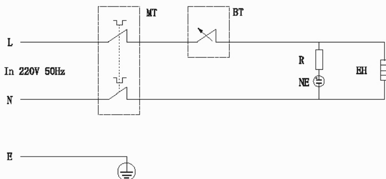
电气原理图
