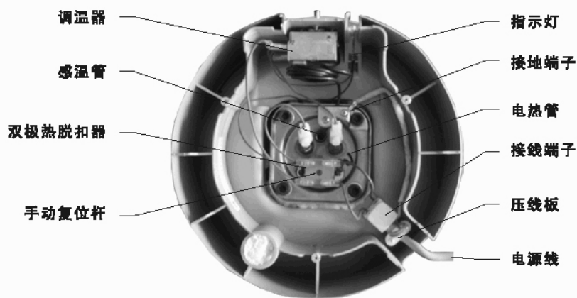
接线图
