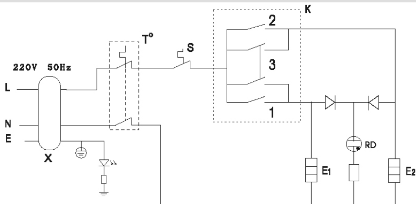
电气原理图
